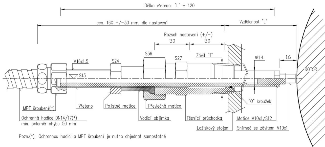
Obr.1: Náskres držáku P6492
