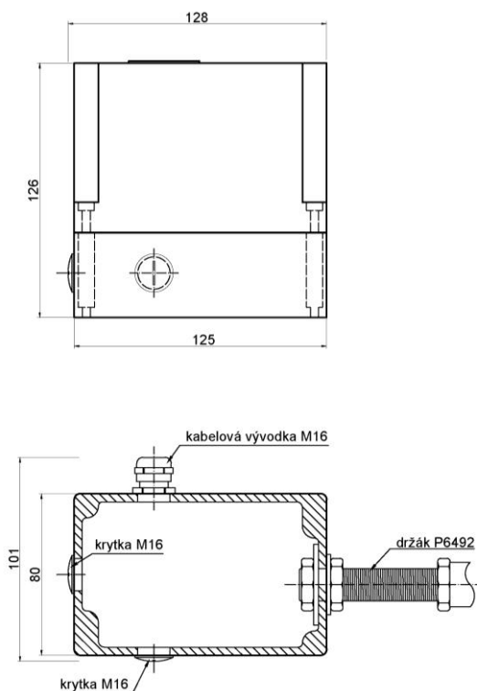
Obr.2: P6492 s ochranným boxem pro převodník (volitelné)
