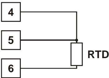
Pt100-Fühler in 3-Leiterschaltung
