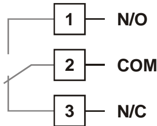
Bild 21 - Options-Steckplatz 1 - Relais-Modul
