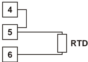
Pt100-Fühler in 2-Leiterschaltung
