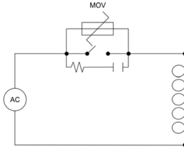
Bild 8 - Störunterdrückung bei Kontakten
